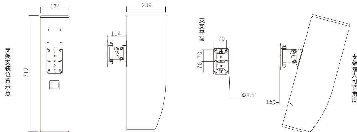
铁支架安装示意图
