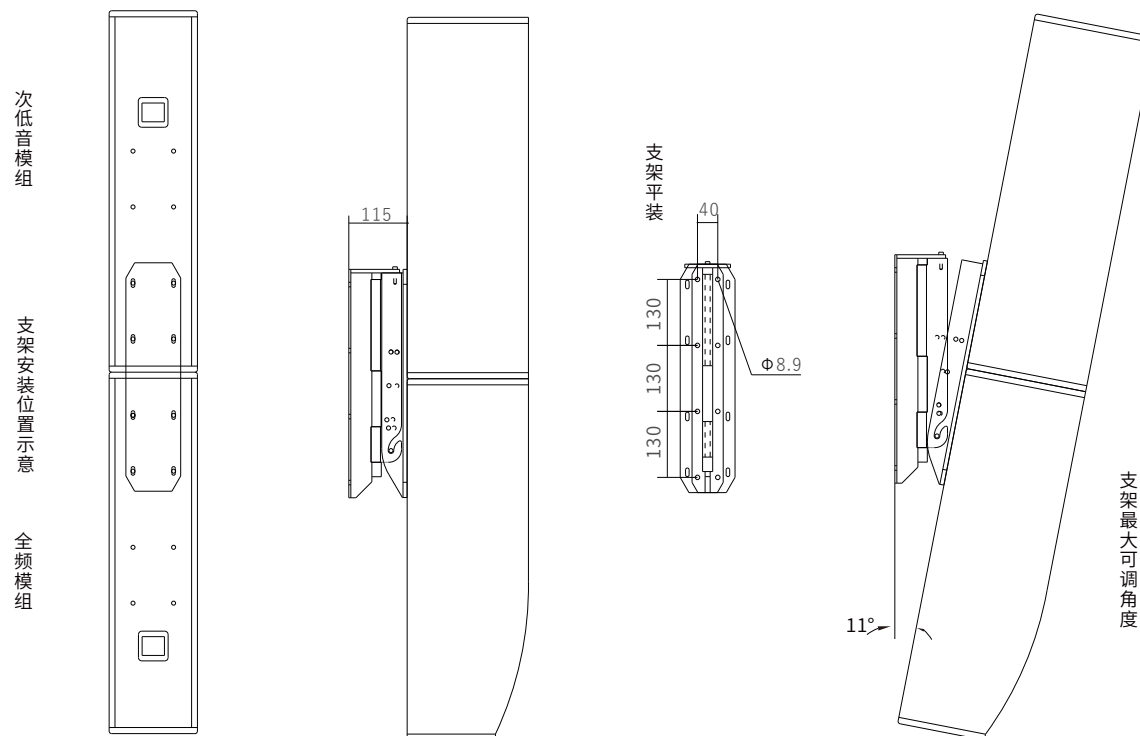
组合支架安装示意图
